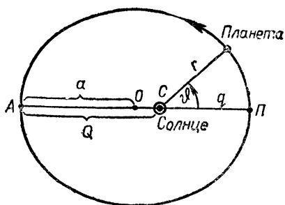
Рис. 4. Эллиптическая орбита
