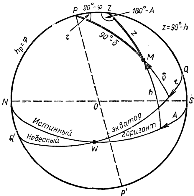
Рис. 3. Параллактический треугольник
